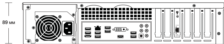
Вид сзади
