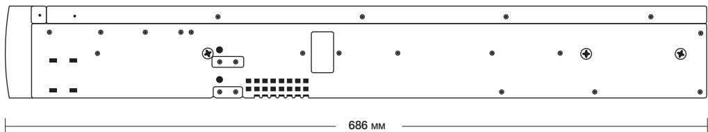
Вид сбоку
